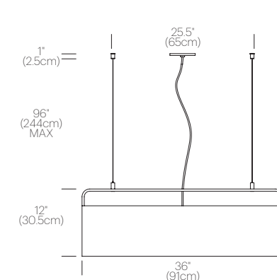
TUBE TOP PENDANT 36
